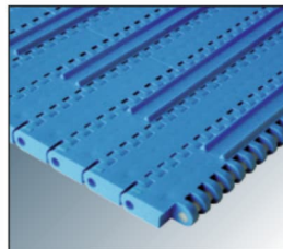
Powierzchnia z nieprzylegającymi poprzecznymi krawędziami
