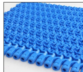
Prześwit 26% Grubość 9 mm + sworznie Powierzchnia typu grill ze sworzniami bez przylegania
