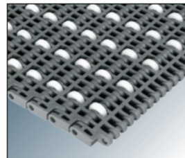
Powierzchnia z rolkami (fi 15 mm) do akumulacji produktu
