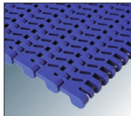
Prześwit 30% Grubość 11 mm Owalne otwory [9.5 x 3] mm
