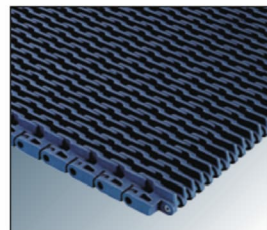
Prześwit 30% Grubość 15 mm Transfer z płytą palcową
