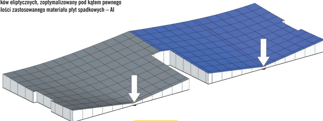
Model 3D – spadki eliptyczne: strzałki wskazują miejsca lokalizacji wpustów dachowych
