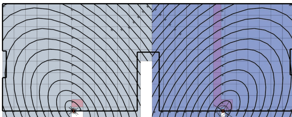
Projekt odwodnienia i spadków eliptycznych, zoptymalizowany pod kątem pewnego odprowadzenia wody oraz ilości zastosowanego materiału płyt spadkowych – Al
