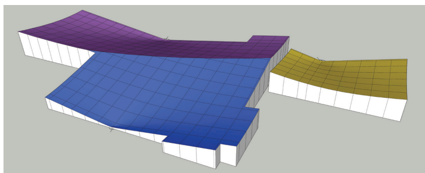
Rys. 5. SPADKI ELIPTYCZNE – wizualizacja 3D spadków do wpustów
