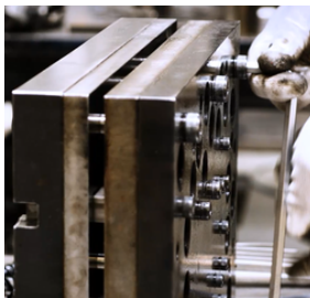
Produkcja tłoczników
