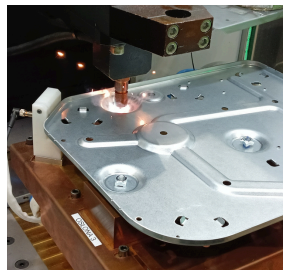
Zgrzewanie
