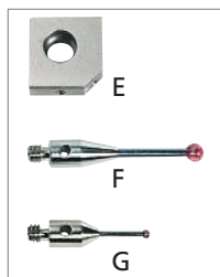
3xM2 płytki czujnika E ER-009899 ø 2 mm F ER-003350 ø 1 mm G ER-003358 dla 2D czujnik krawędziowy
