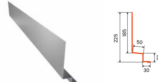
obróbka łącząca boczna PHR
