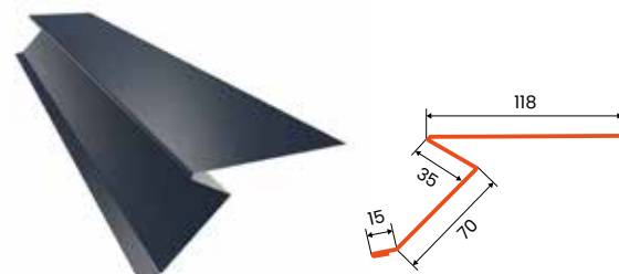
pas nadrynnowy startowy PHR
