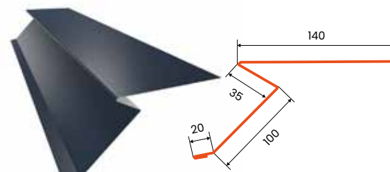
pas nadrynnowy startowy duży PHR
