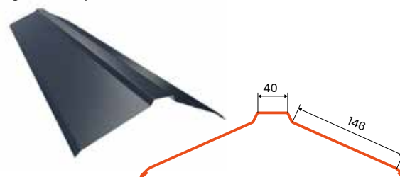
gqsior trapez PHR
