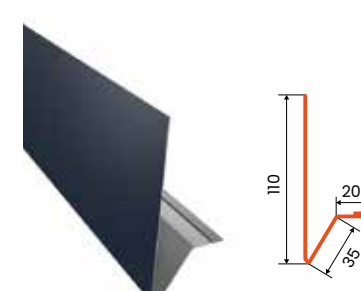
pas zaciągowy PHR
