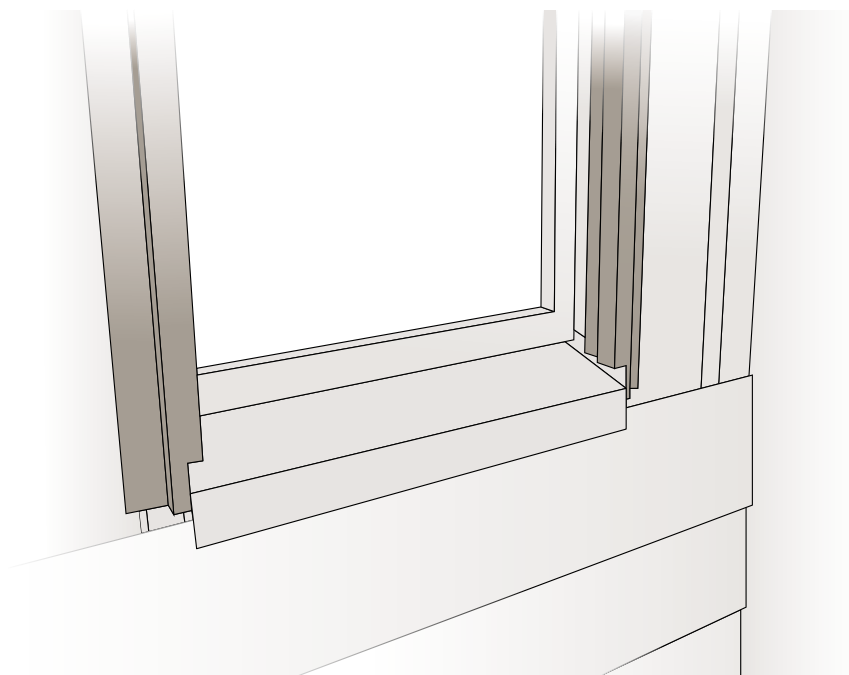
Mocowanie zewnętrznych profili okiennych (asymetrycznych) do boków okna.
