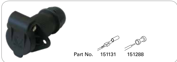
3P/6-24V Socket (Similar DIN 9680)
