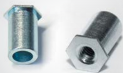
TULEJKA PRZELOTOWA M2-M5 T-SO, T-SOS, T-SO4, T-SOA
