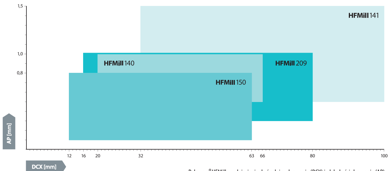
Polcomm® HFMill w odniesieniu do średnicy skrawania (DCX) i głębokości skrawania (AP) Polcomm® HFMill Solutions in relation to cutting diameter (DCX) and depth of cut (AP)
