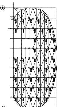
ROZMIESZCZENIE ELEMENTÓW MOCOWANIA PASADY W OSI G07
