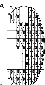
ROZMIESZCZENIE ELEMENTÓW MOCOWANIA FASADY W OSI G29
