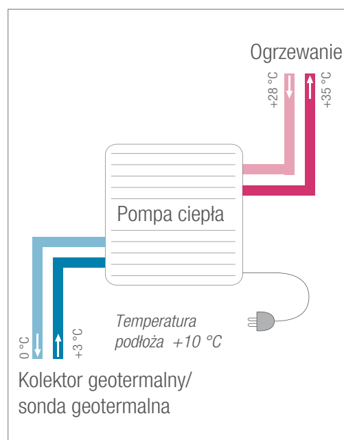
Zasada działania pompy ciepła
