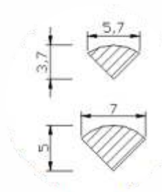
Dysza okrągła o średnicy wylotu \varnothing 4mm z gwintem M10 Nr zamów. 5410186 RD4
